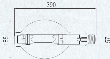
SK20NR-C
