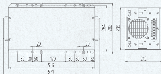
KSL-402B KSL-402HB
