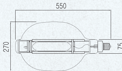
SK30NR-C
